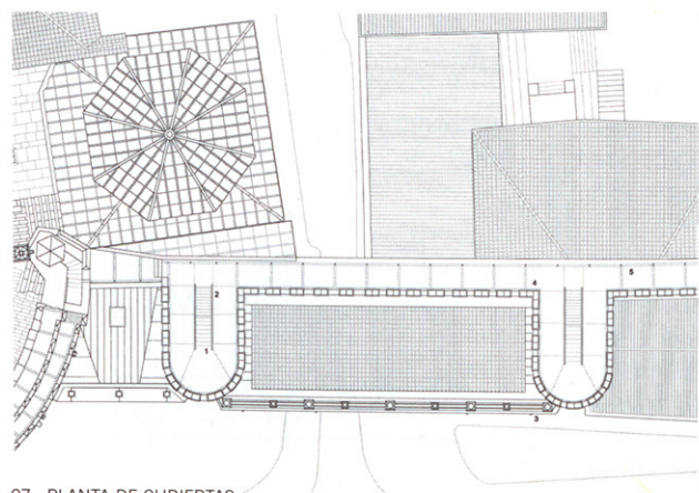
07 · PLANTA DE CUBIERTAS
